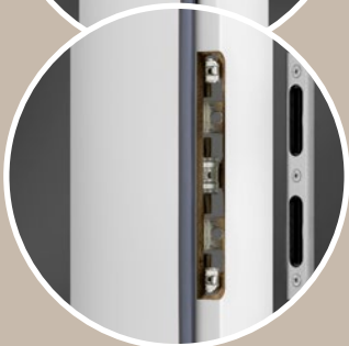
Sicherheitsschließblech fest im Türfutter verschraubt
